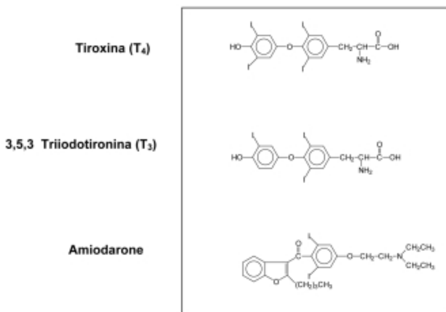
Figura 1. Formule chimiche degli ormoni tiroidei e dell'amiodarone.
