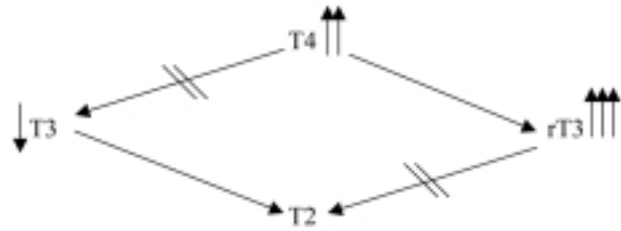
Figura 2. Modificazioni del metabolismo degli ormoni tiroidei indotte dall'amiodarone.
