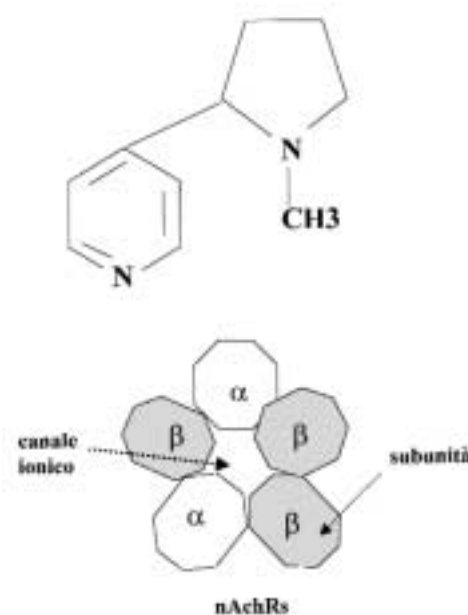
Figura 1. Schema della struttura molecolare della nicotina e dei suoi recettori colinergici (nAChRs).
