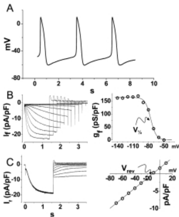
Figura 2. Proprietà della corrente I_f nel nodo senoatriale. A: potenziali d'azione spontanei registrati in un miocita, mediante la tecnica del "patch-clamp"; B: in "voltage-clamp", in seguito all'imposizione di gradini iperpolarizzanti a valori via via più negativi, è possibile registrare una corrente in ingresso che si attiva nell'arco di alcuni secondi; il grafico a destra mostra la tipica relazione corrente-voltaggio, in cui è indicato il potenziale di metà attivazione della corrente ( V_{1/2} ) che in questo caso è intorno a -70 mV; C: l'analisi delle "tail currents", che rappresentano la deattivazione della corrente, consente di calcolare il potenziale di inversione ( V_{rev} ) di I_f che è di circa -15 mV, come atteso per un canale con permeabilità mista a ioni di sodio e potassio.
