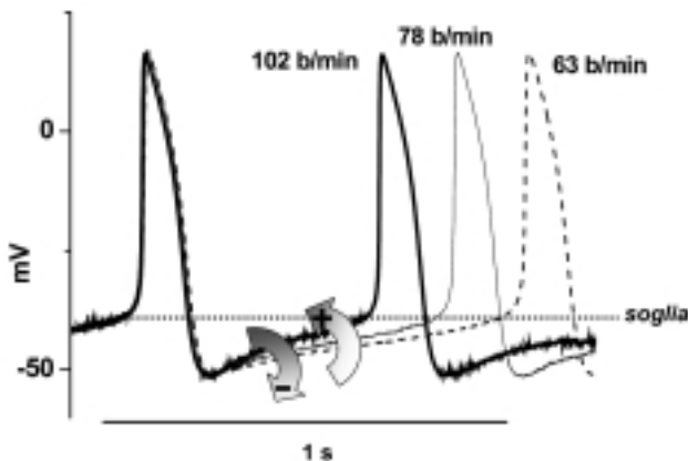
Figura 3. La regolazione della pendenza della depolarizzazione diastolica, da parte delle catecolamine (+) e dell'acetilcolina (-), determina la frequenza spontanea nelle cellule pacemaker.
