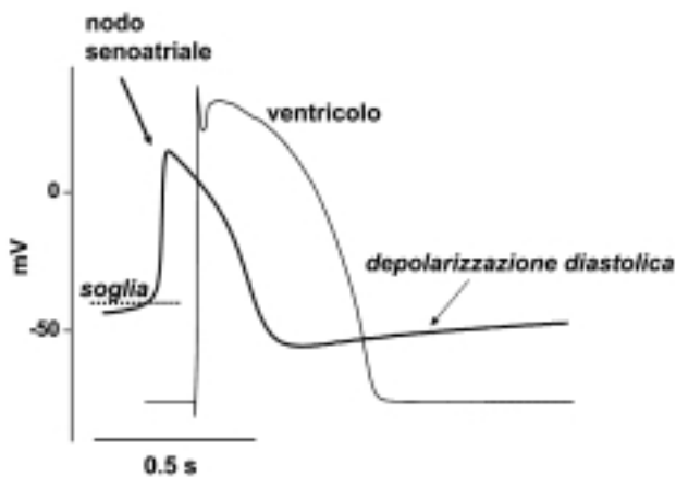
Figura 1. Tipico profilo del potenziale d'azione in una cellula del nodo senoatriale e in un miocita ventricolare.
