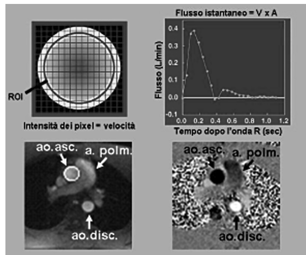
Figura 2. Calcolo della portata cardiaca anterograda del ventricolo sinistro utilizzando la tecnica phase-contrast velocity mapping . In alto a sinistra: schema della sezione trasversale di un vaso il cui contorno endocardico è delimitato da una regione di interesse (ROI), all'interno della quale ad ogni pixel corrisponde un valore di velocità. In alto a destra: moltiplicando l'area di sezione del vaso per la velocità media di flusso si ottiene il flusso istantaneo, il cui andamento durante il ciclo cardiaco è rappresentato dalla curva flusso/tempo ottenuta automaticamente dal software di analisi. In basso a sinistra: il lume dell'aorta ascendente è delimitato da una ROI (in bianco). In basso a destra: la stessa immagine è visualizzata in modalità phase-contrast (il lume aortico appare nero).
