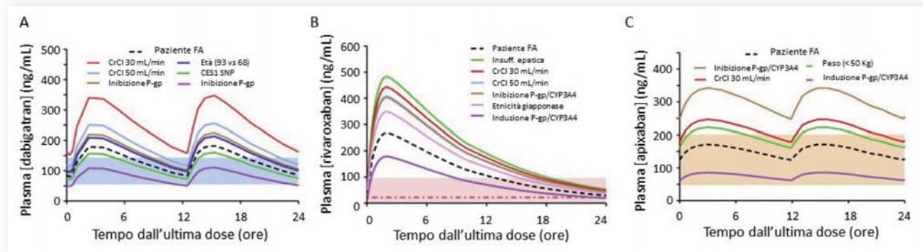
Figura 5. Profilo concentrazione-tempo dei nuovi anticoagulanti orali in base alla funzionalità renale ed epatica, alla co-somministrazione di inibitori ed induttori di P-gp e CYP3A4.
